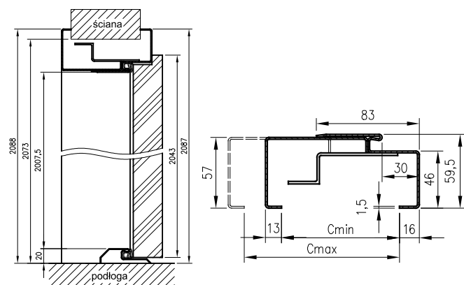
ościeżnica stalowa regulowana
