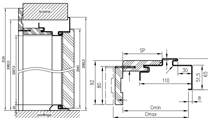
ościeżnica stalowa hybrydowa
