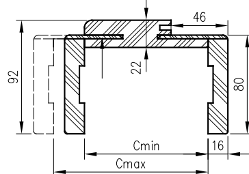
Ościeżnica Regulowana Bezprzylgowa z T80
