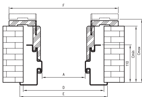
Ościeżnica drewniana do drzwi Athos z progiem stałym
