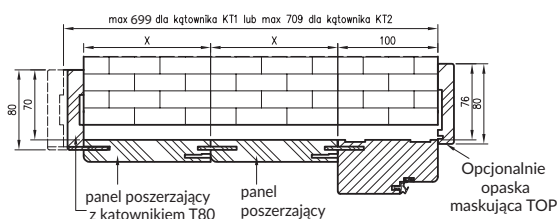
Wariant z dwoma panelami poszerzającymi
