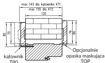
Wariant z kątownikiem KT1 lub KT2
