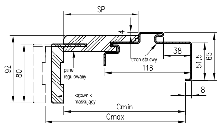
Wymiary OSH do drzwi Athos
