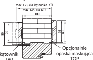
Wariant z kątownikiem KT1 lub KT2
