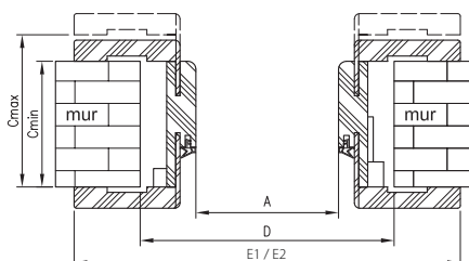
Ościeżnica Regulowana Bezprzylgowa z T63
