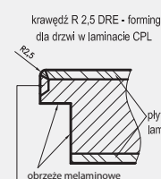
krawędź R 2,5 DRE - forming dla drzwi w laminacie CPL
