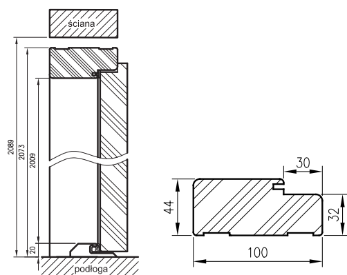
ościeżnica prosta MDF
