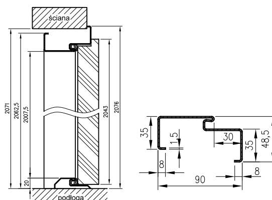
ościeżnica stalowa stała
