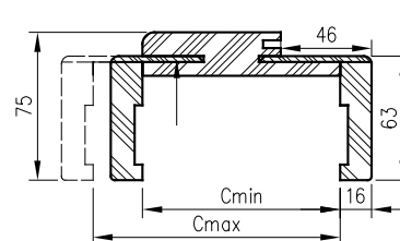
Ościeżnica Regulowana Bezprzylgowa z T63
