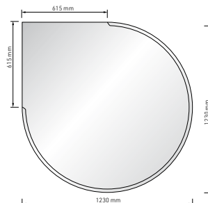
Tropfenform (bei brennbaren Böden)
